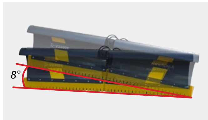
8° kallistuskulma
